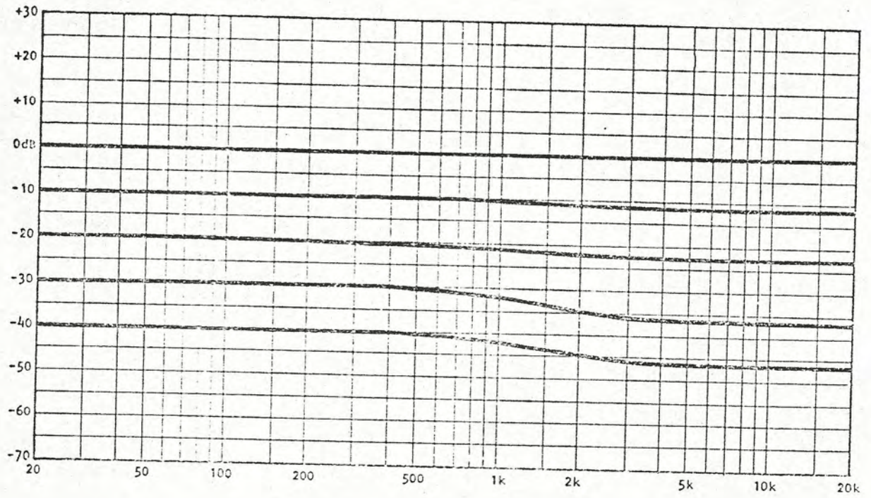
Fig. 3-3, HISS - 6dB
