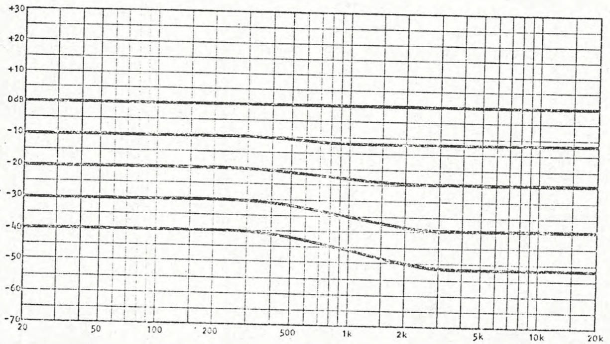
Fig. 3-4, HISS - 12dB
