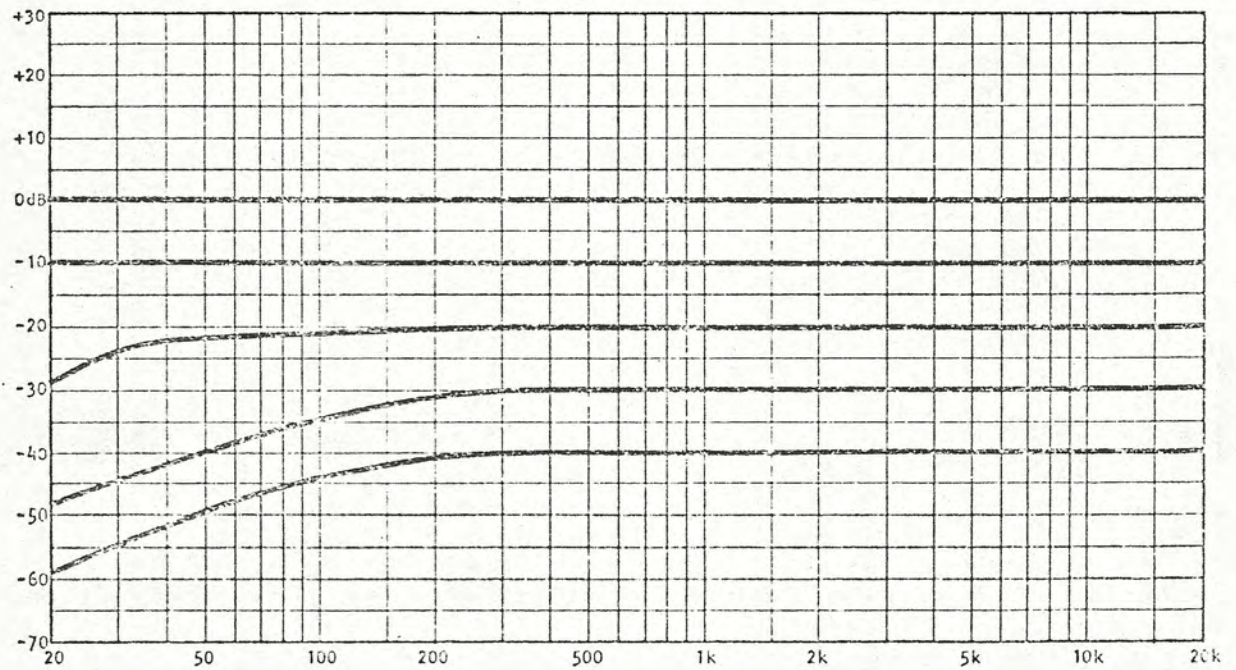
Fig. 3-2, RUMBLE - 13dB
