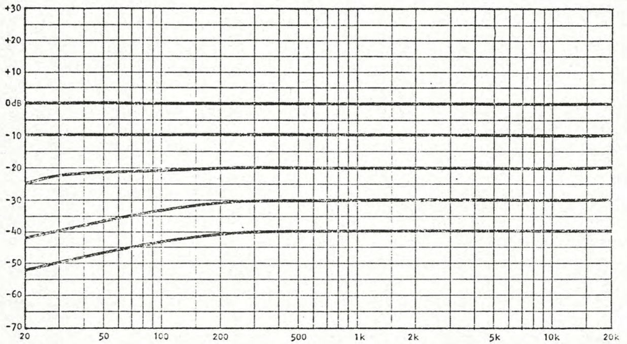
Fig. 3-1, RUMBLE - 12dB
