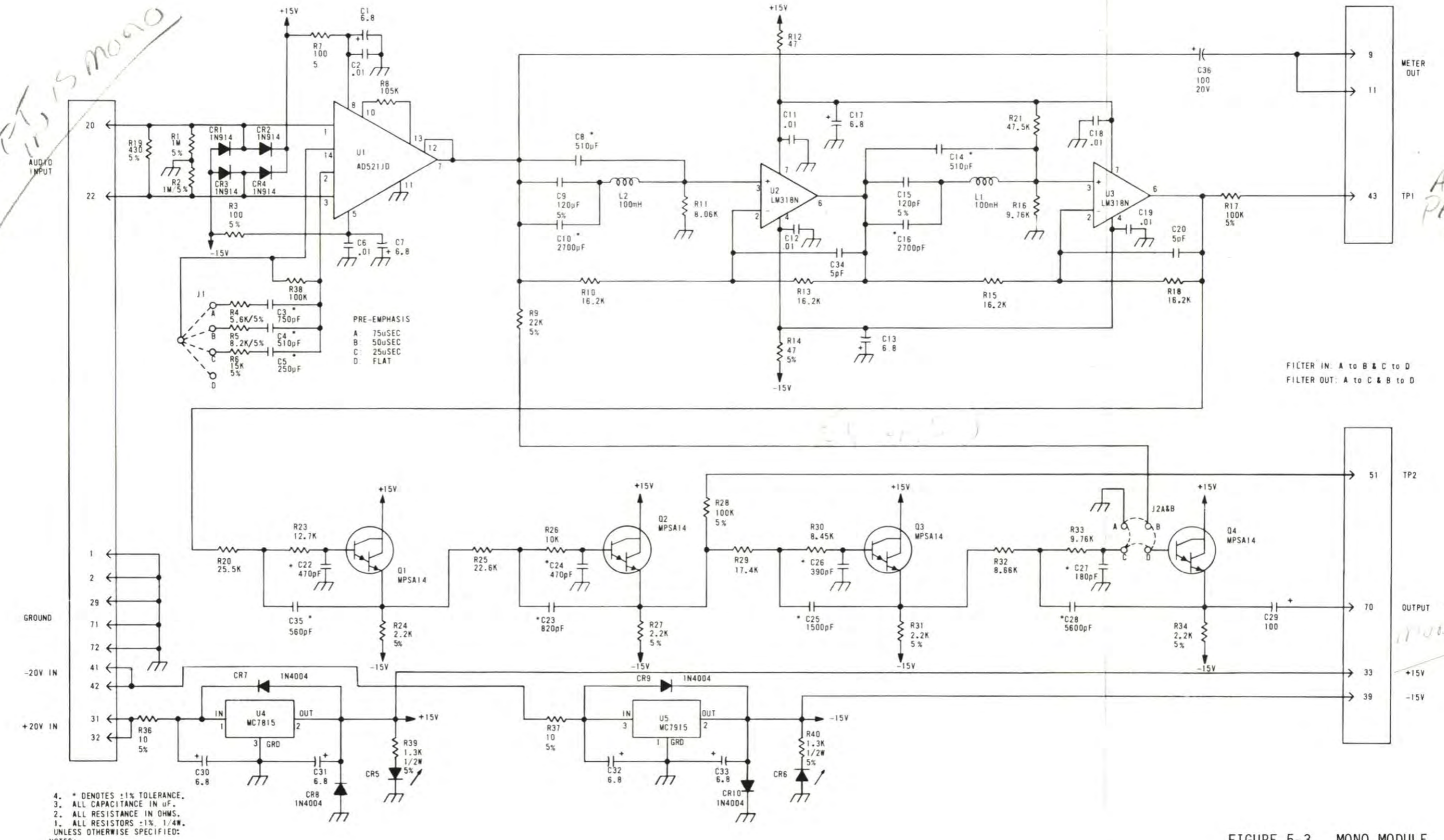
FIGURE 5-3. MONO MODULE SCHEMATIC 843 1703 001
